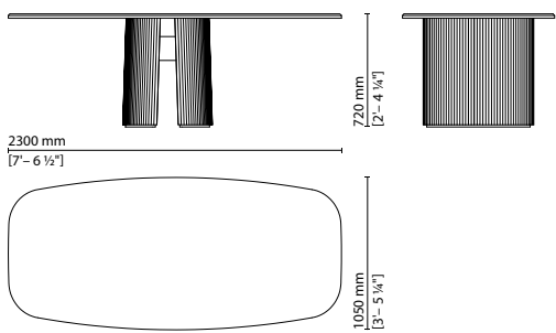
055203 — Dining table
