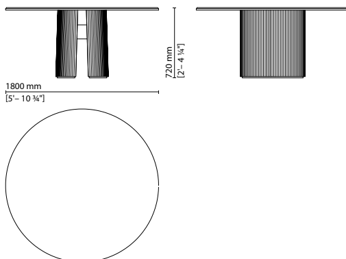
055203 — Dining table
