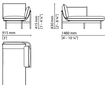
047006 — Right chaise longue
