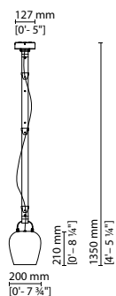
703 901 / 703 902 — Bells
