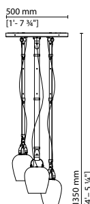
703 903 / 703 904 — Bells 3 pz
