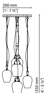
703 905 / 703 906 — Bells 5 pz
